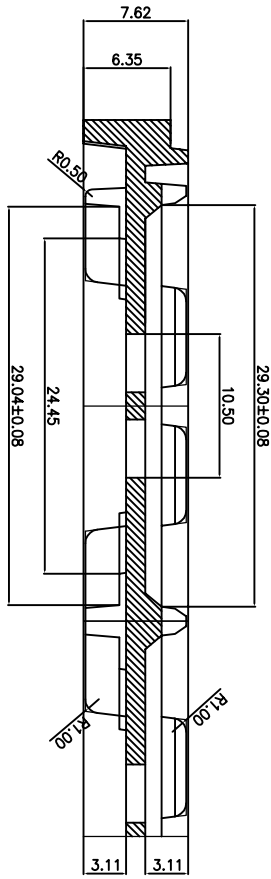
SECTION "A-A" (SCALE: 4/1)
