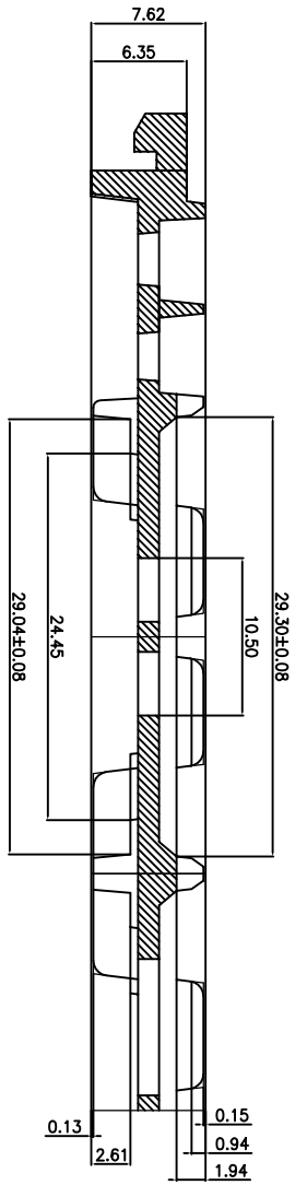
SECTION "A-A" (SCALE: 4/1)
